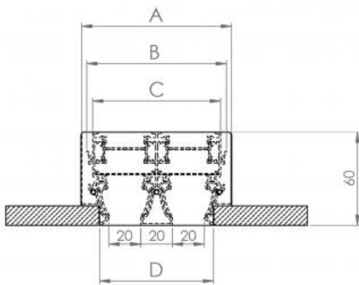
EDLH-FA 2 feritoie 20 mm EDLHB-FA 2 feritoie 20 mm
