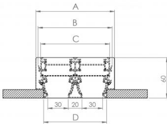
EDLH-FB 2 feritoie 30 mm EDLHB-FB 2 feritoie 30 mm
