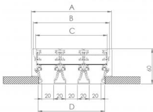
EDLH-FA 3 feritoie 20 mm EDLHB-FA 3 feritoie 20 mm
