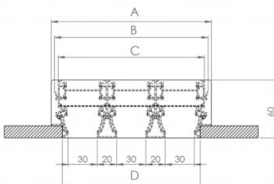
EDLH-FB 3 feritoie 30 mm EDLHB-FB 3 feritoie 30 mm
